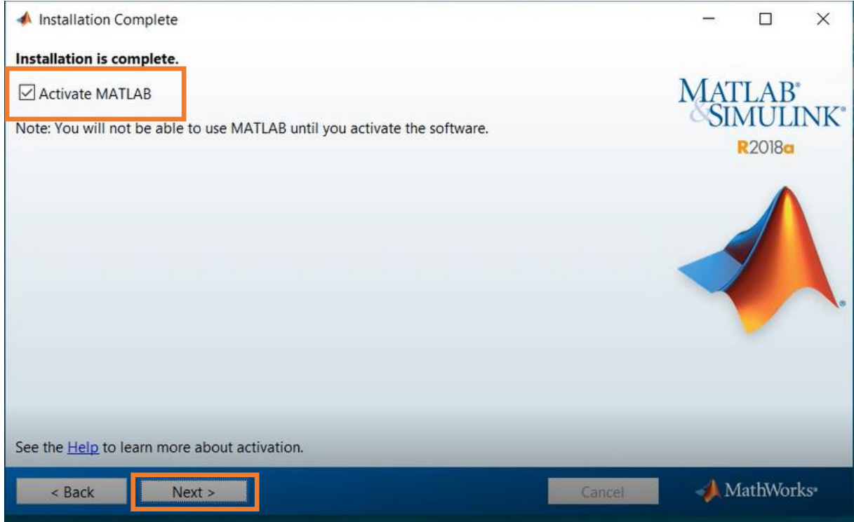
Şekil 15: Aktivasyon ekranı
