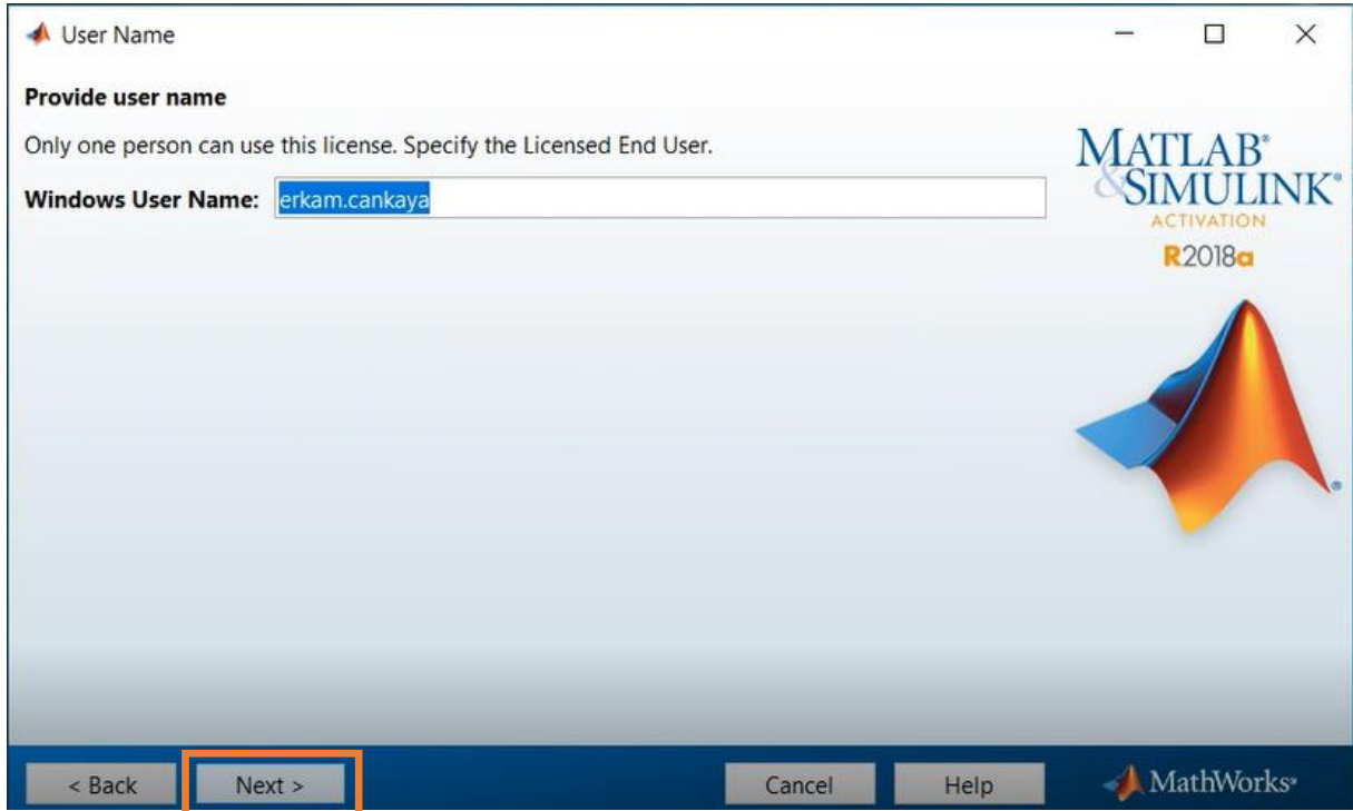
Şekil 17: Kişi Aktivasyonu
