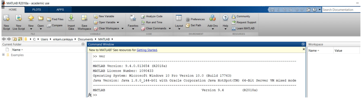
Şekil 20: MATLAB'in açılması
