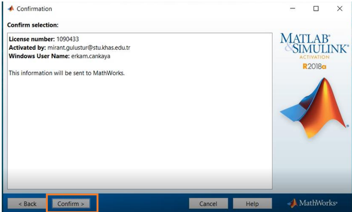
Şekil 18: Doğrulanma Aşaması
