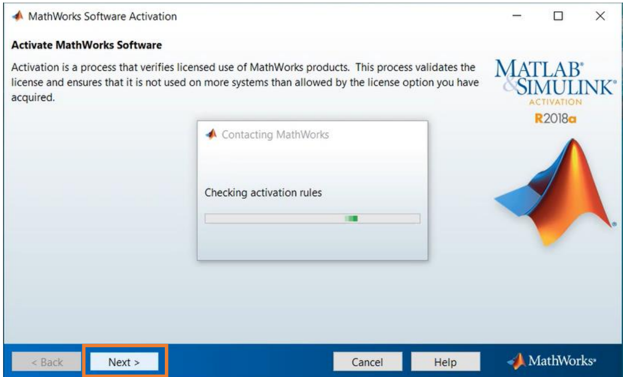
Şekil 16: Aktivasyon süreci
